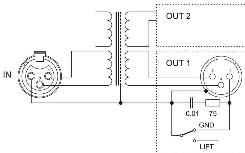
Рис. 1. Функциональная схема трансформаторного распределителя DS-412ASTM
