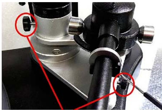
Ослабьте два винта для настройки VTA
