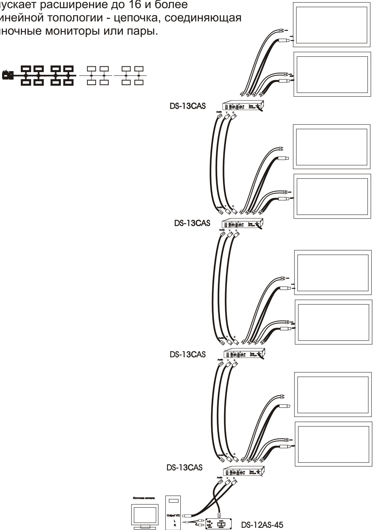
Схема на 8 мониторов, вариант линейной цепочки
