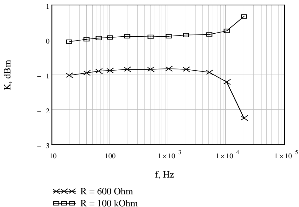
Рис. 6. Типовая зависимость суммарного коэффициента передачи от частоты входного сигнала и сопротивления нагрузки.
