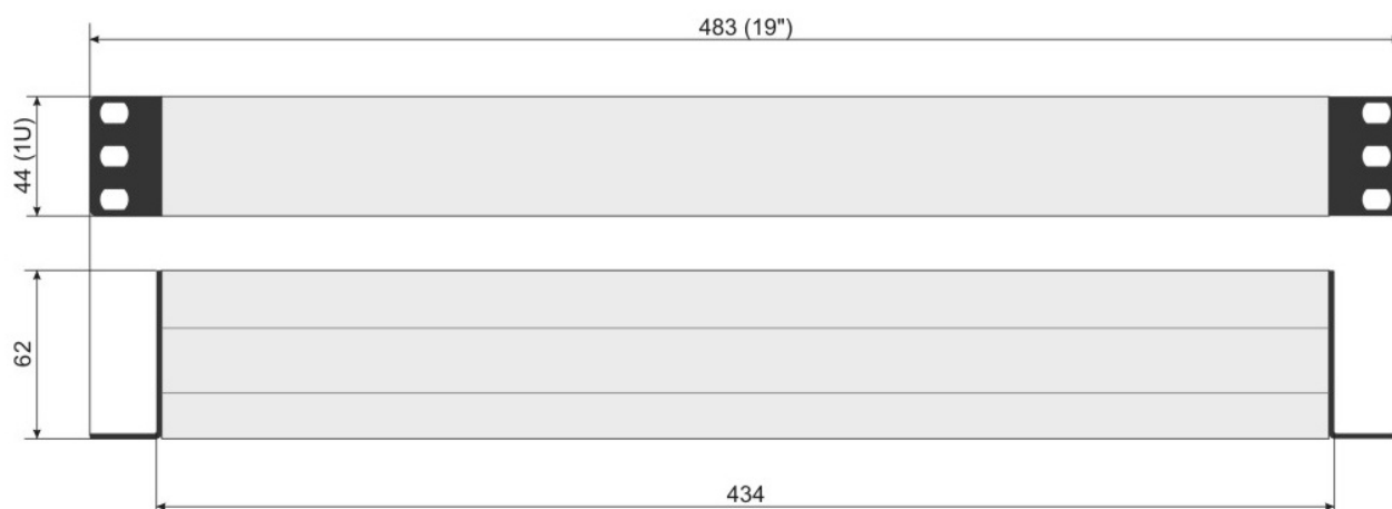
Габаритные размеры TR-81AS(M)
