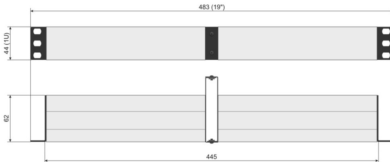
Парное исполнение для установки в приборную стойку, шириной 19" (483 мм) – TR-41AS(M)-3
