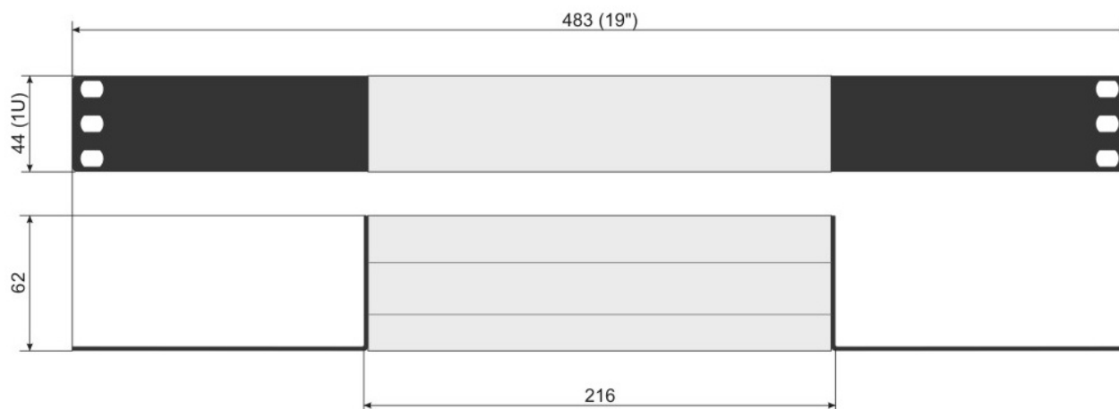
Исполнение для установки в приборную стойку, шириной 19" (483 мм) – TR-41AS(M)-2
