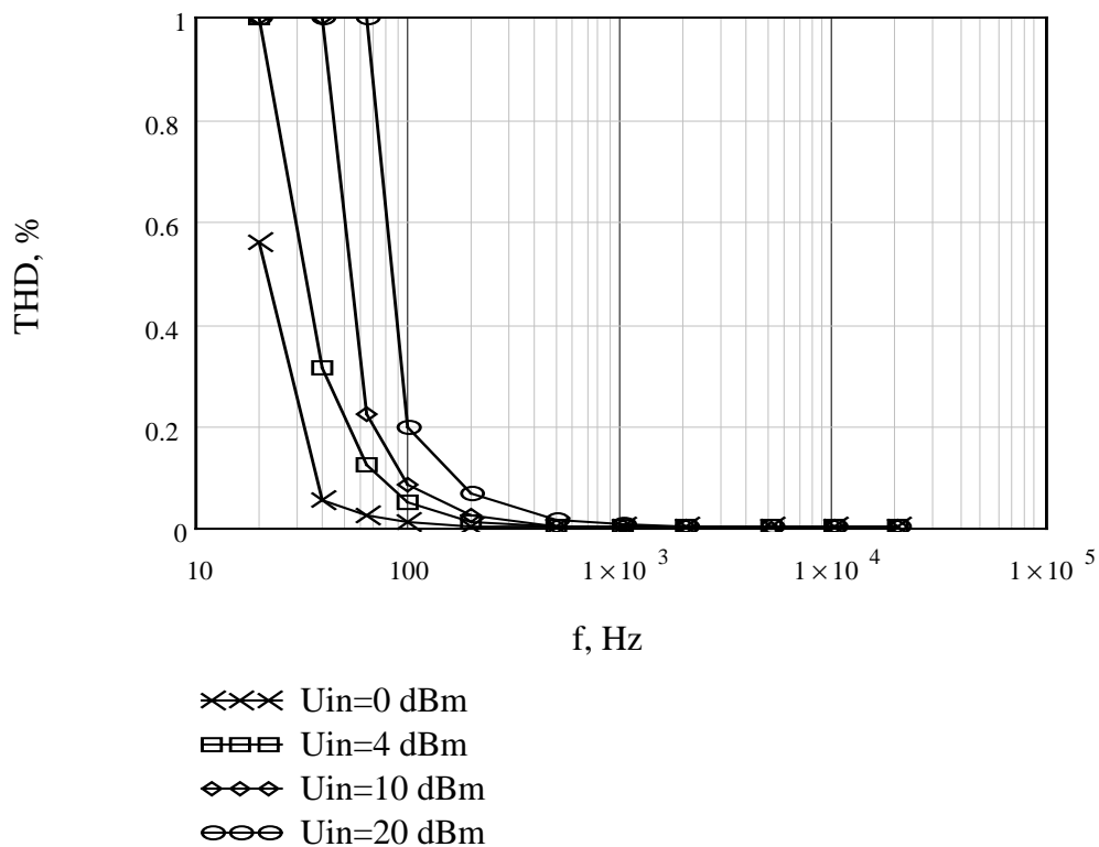
Рис. 5. Типовая зависимость суммарного коэффициента нелинейных искажений от частоты и уровня входного сигнала.
