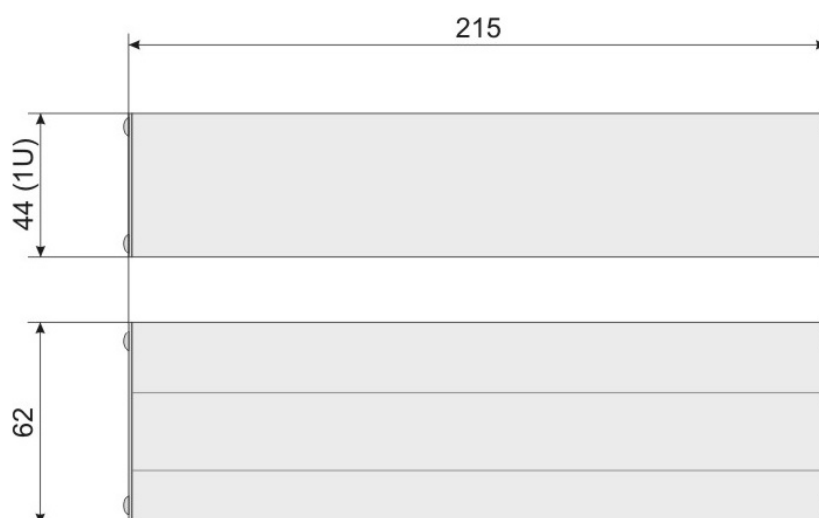
Настольное исполнение TR-41AS(M)
