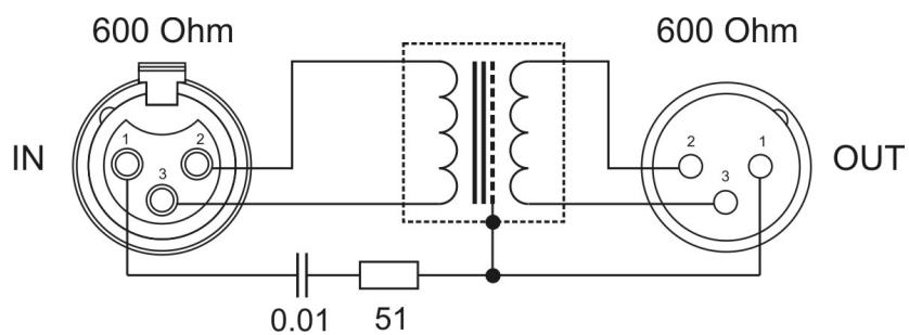
Рис. 2. Функциональная схема одного канала прибора TR-41ASM (TR-81ASM) с защитным экраном.
