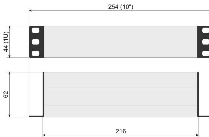
Исполнение для установки в приборную стойку, шириной 10" (254 мм) – TR-41AS(M)-1
